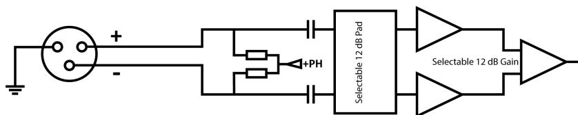
SLXD3+
